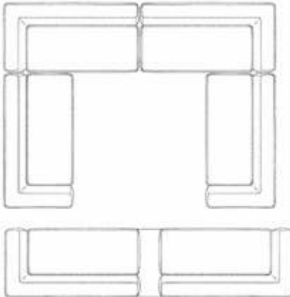
ORO 02 | İkili kanepi | double W 180 cm. D 73 cm. H 71 cm.
