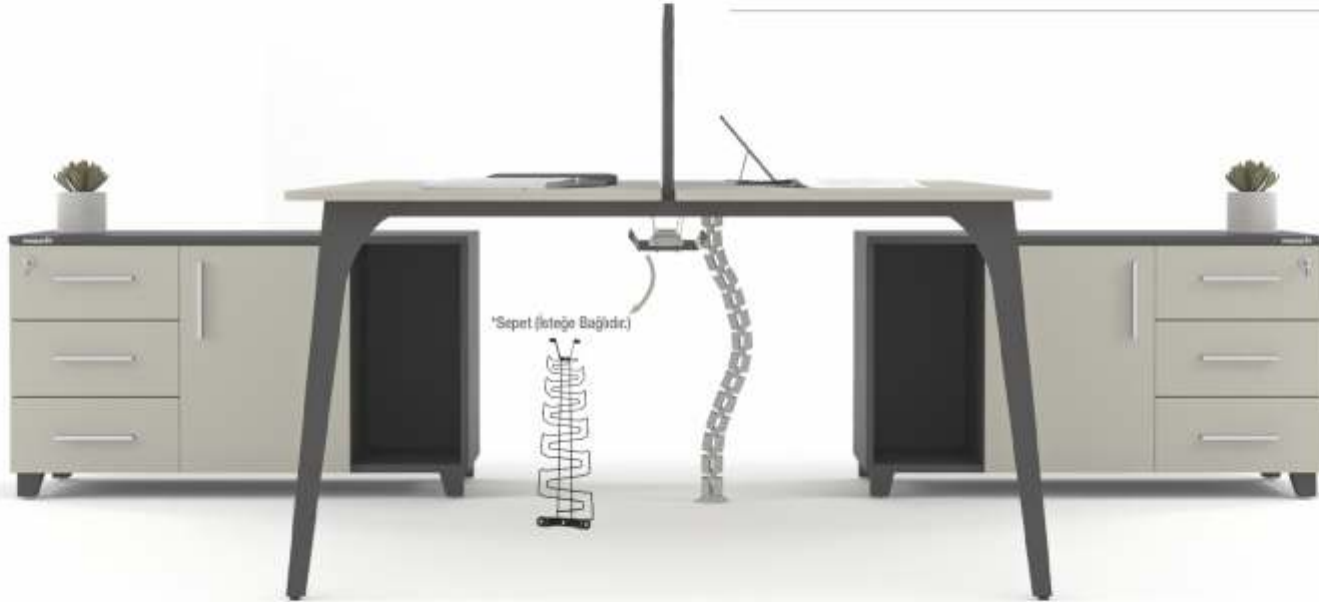
CWO 15 İkili çalışma masası double working desk L 180 cm. D 142 cm. H 110 cm. CET 01 Etajer (2 adet) etagere L 80 cm. D 50 cm. H 75 cm. OKK 01 Omurga kablo kanalı
