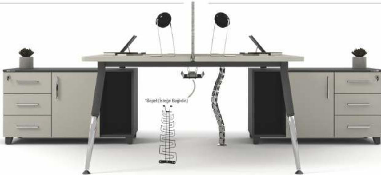
BWR 15 İkili çalışma masası double working desk L 180 cm. D 142 cm. H 110 cm. KSO 02 01 Keson(2 adet) pedestal L 40 cm. D 47 cm. H 62 cm.
